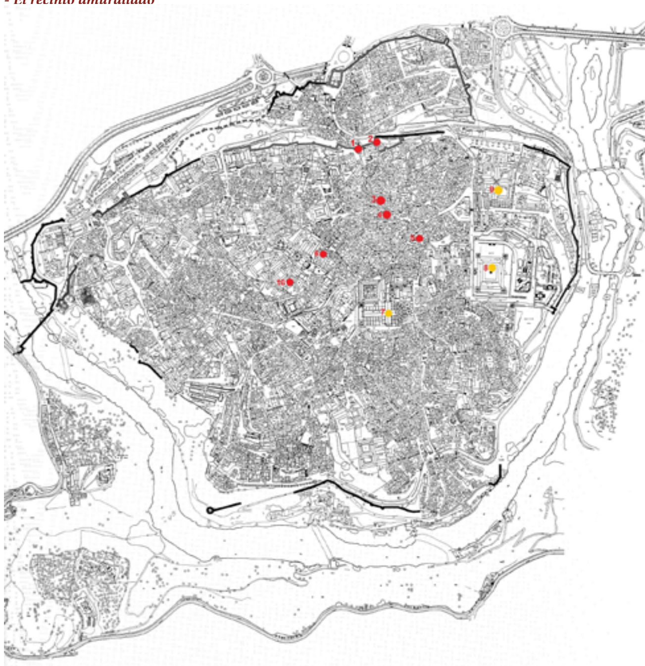
Fig. 2. Toledo, situación de espacios urbanos intramuros. 1. Acceso norte (Bab-al-Mardúm); 2. Torre romana de la Puerta del Sol; 3. Área del foro; 4. Cueva de Hércules; 5. Termas; 6. Cta. de Portugueses; 7. Catedral medieval; 8. Alcázar; 9. Santa Fé ; Palatium visigodo?; 10. Madre de Dios. Elaboración propia. Base: Las murallas de Toledo , Madrid, Fundación Caja Madrid, 2004, p.167.
