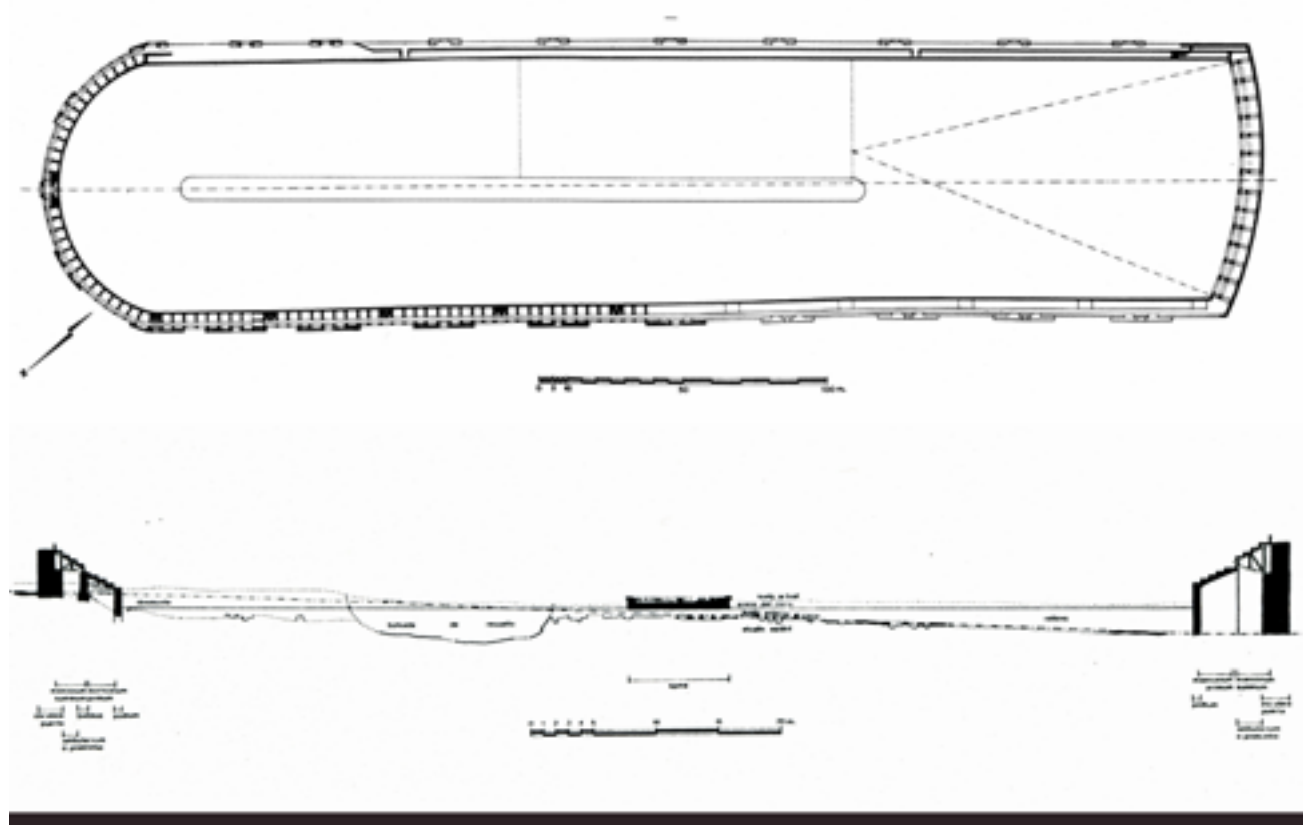
Fig. 8. Planimetría y sección del circo romano de Toledo (de Sánchez Palencia y Sainz, "El circo romano").
