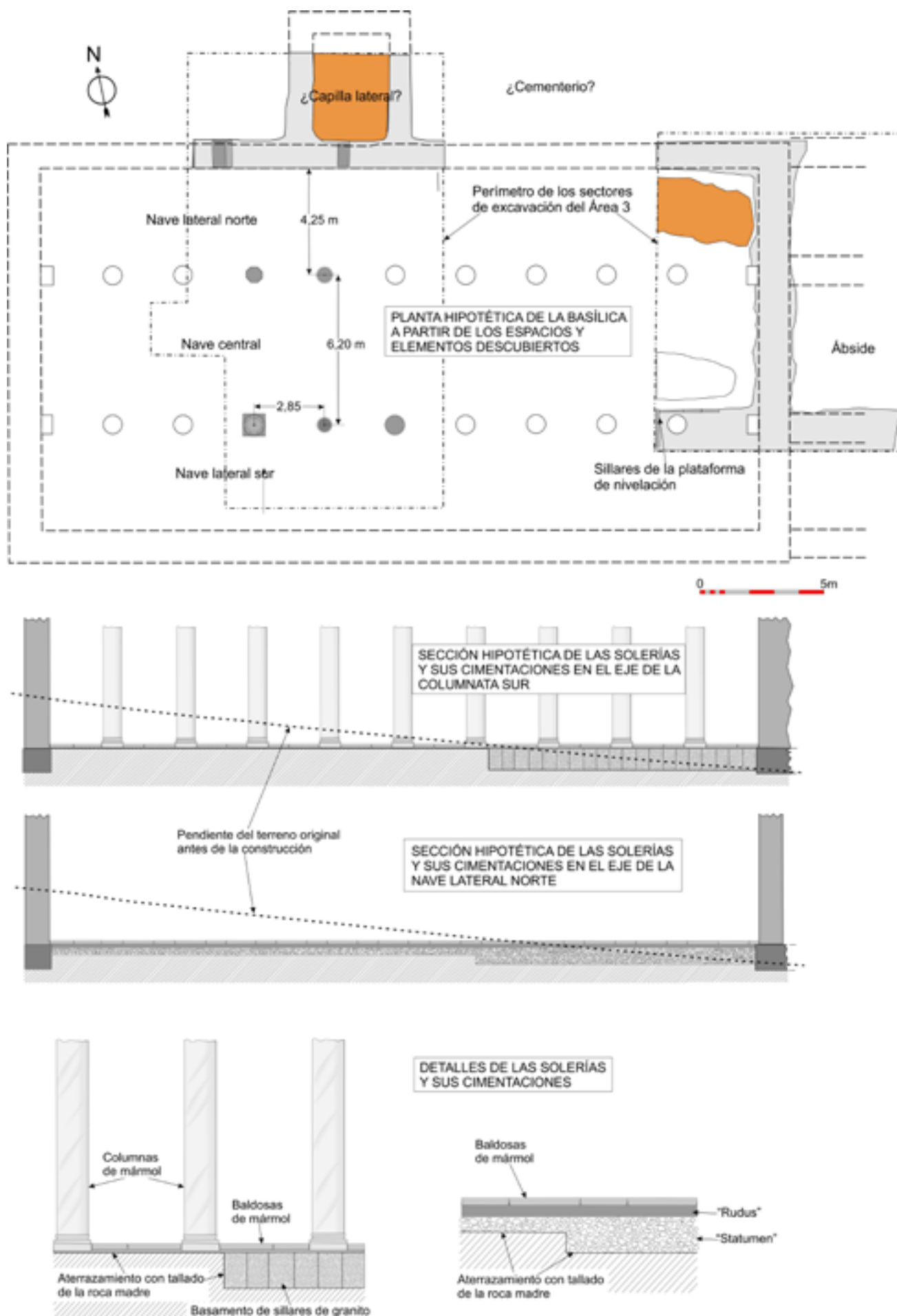
Fig. 7. Planta y secciones hipotéticas del edificio de la basílica (según J.M. Rojas, A. Vicente y Ch. Eger).
