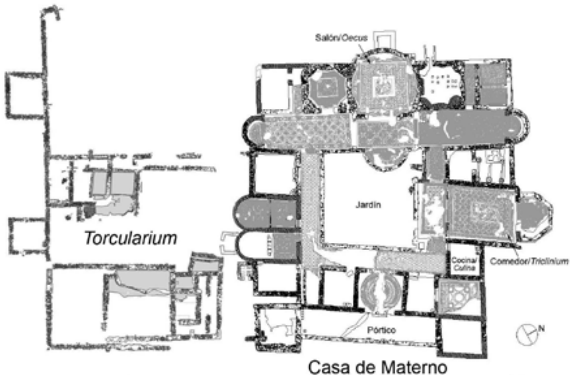
Fig. 6. Carranque, villa de Materno. Dibujo: Equipo de investigación de Carranque. De V. García Entero, et aliae, "La producción de aceite y vino en el interior peninsular. El ejemplo de la villa de Carranque (Toledo)", Anales de Prehistoria y Arqueología , 27-28 (2011-2012), p. 166, fig. 5.
